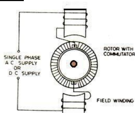
Fig. 7.17: Universal motor
